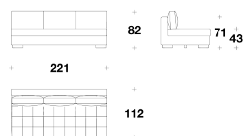
SHT (E3C) ELEMENTO 3 POSTI CENTRALE / 3 SEATER CENTRAL ELEMENT 221x112x82H. - H.S.43cm 87x44x32 1/3H. - H.S.17"
