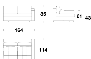
SHT (E2DB) - SHT (E2SB) ELEMENTO 2 POSTI CON BRACCIOLO DX O SX / 2 SEATER ELEMENT WITH RIGHT OR LEFT ARMREST 164x114x85H. - H.A.61 - H.S.43cm 64 2/3x45x33 1/3H. - H.A.24 - H.S.17"
