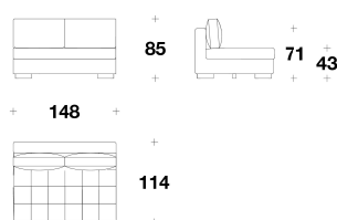
SHT (E2C) ELEMENTO 2 POSTI CENTRALE / 2 SEATER CENTRAL ELEMENT 148x114x85H. - H.S.43cm 58 1/3x45x33 1/3H. - H.S.17"
