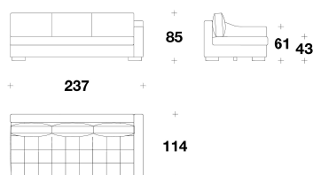
SHT (E3DB) - SHT (E3SB) ELEMENTO 3 POSTI CON BRACCIOLO DX O SX / 3 SEATER ELEMENT WITH RIGHT OR LEFT ARMREST 237x114x85H. - H.A.61 - H.S.43cm 93 1/3x45x33 1/3H. - H.A.24 - H.S.17"
